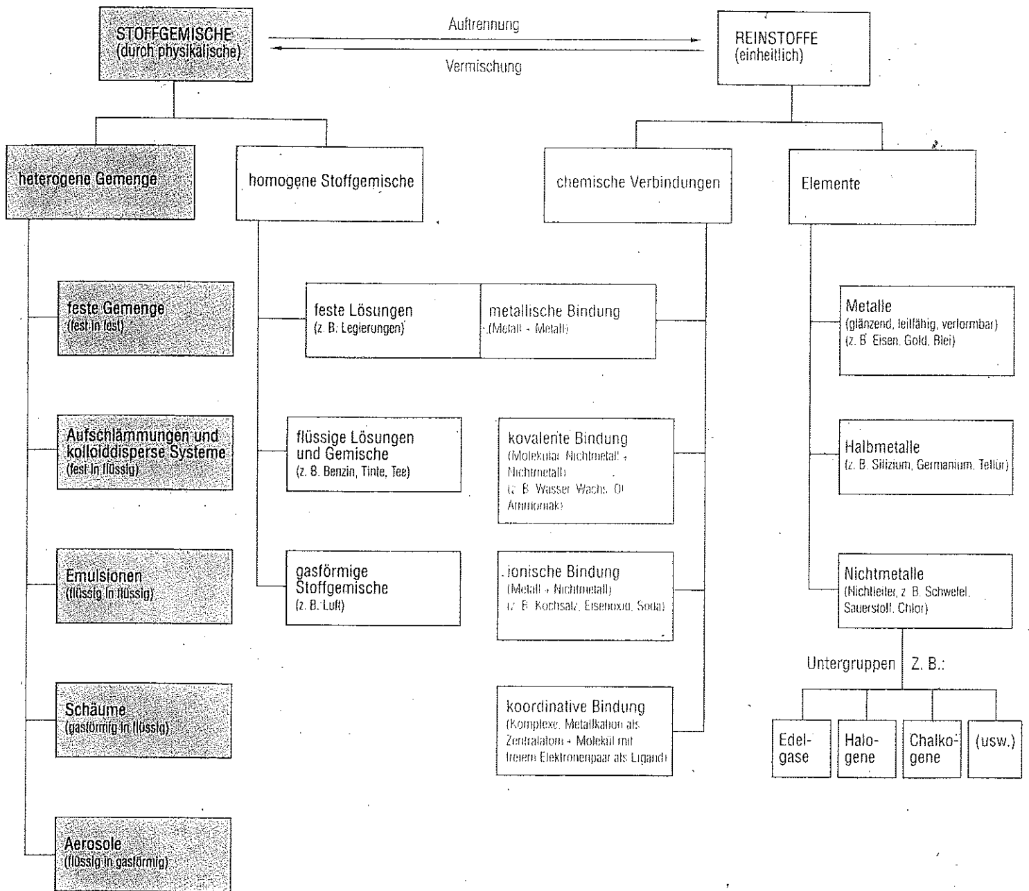
Abb. 1.2.1-3 Einteilung von Materialproben
